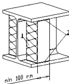
Rys. 2b. Mocowanie klocków klinowych z płyt z wełny mineralnej do elementu stalowego w systemie CONLIT 150 w przypadku wysokości środnika elementu stalowego większej niż 500 mm
