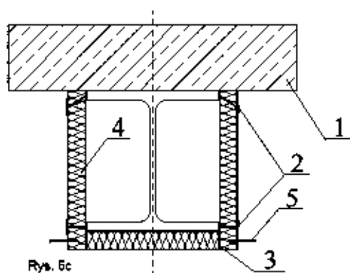
Rys. 5. Trójścienna izolacja ogniochronna elementu stalowego wykonana systemem CONLIT 150, sposobem II – sposoby mocowania izolacji do elementu stalowego
