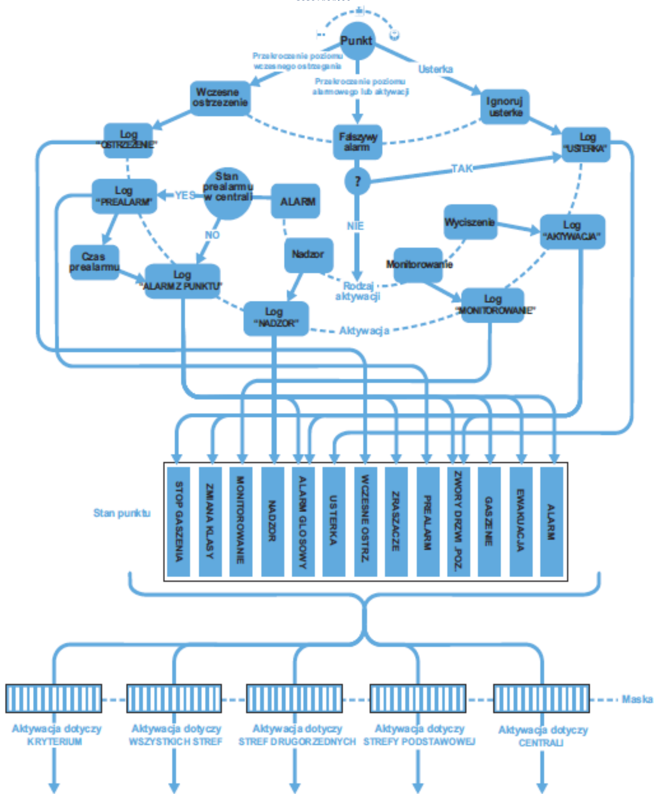
Rysunek 1 - Wejścia: Aktywacja sygnalizacji z punktu
