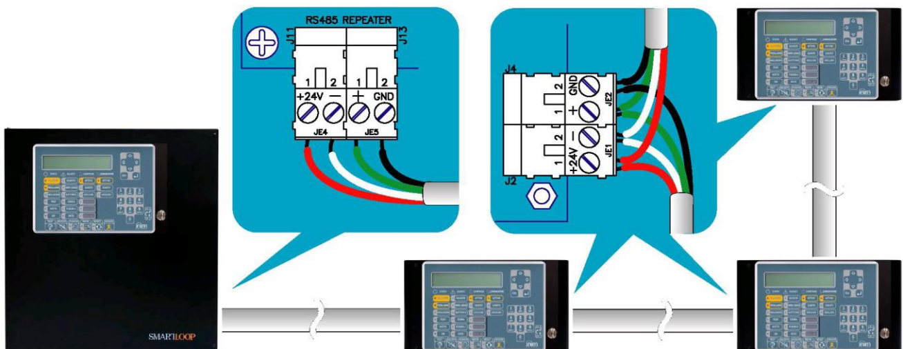
Rysunek 32 - Podłączenie terminali wyniesionych
