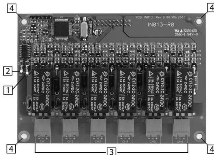
Rysunek 15 - Moduł SmartLoop/INOUT
