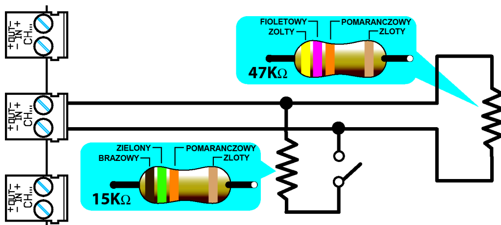
Rysunek 37 - Wejście nadzorowane
