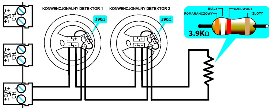
Rysunek 35 - Konwencjonalna linia pożarowa
