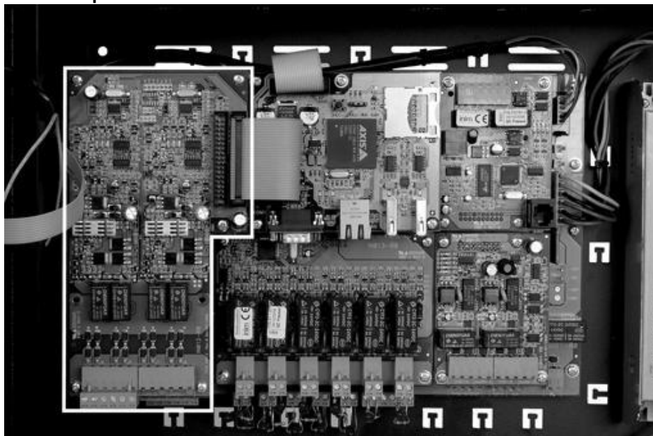
Rysunek 8 - Moduł SmartLoop/2L zamontowany na płycie głównej centrali
