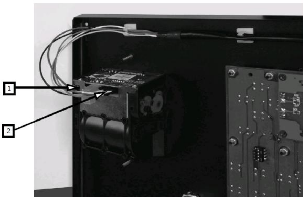
Rysunek 20 - Moduł SmartLoop/PRN (drukarka) zamontowany na płycie czołowej centrali
