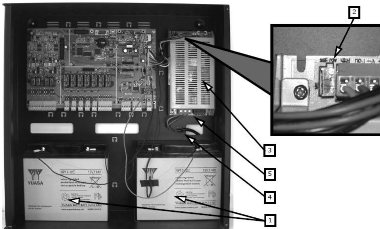
Rysunek 40 - Zasilanie sieciowe, podłączenie akumulatorów i trymer regulacyjny
