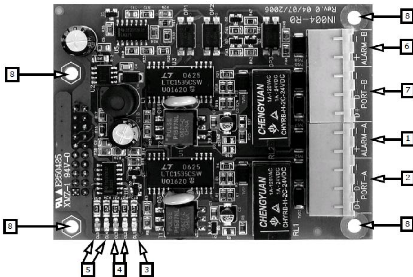
Rysunek 9 - Moduł SmartLoop/NET
