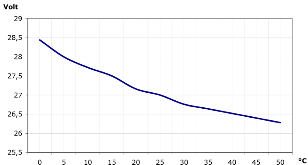
Rysunek 39 - Zależność napięcia ładowania akumulatorów od temperatury
