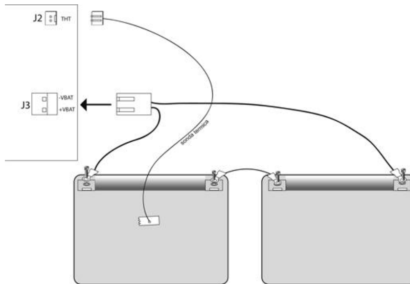
Rysunek 38 - Podłączenie akumulatorów
