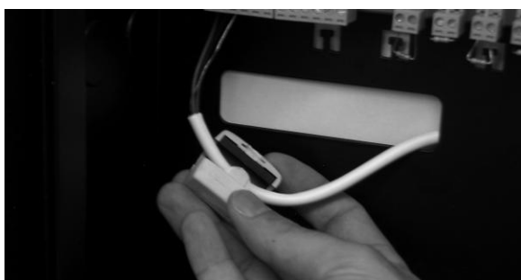
Rysunek 28 – Zakładanie rdzeni ferrytowych na przewody pętli
