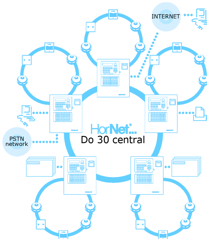
Rysunek 1 - Przykładowa konfiguracja: 5 central w zamkniętej strukturze sieciowej (HorNet)
