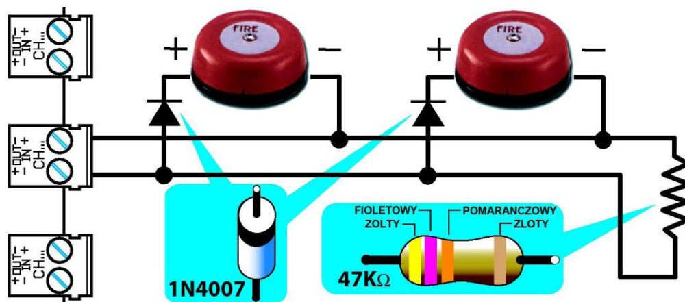
Rysunek 34 - Wyjście nadzorowane NAC
